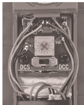
DCC-DCS Schalter
